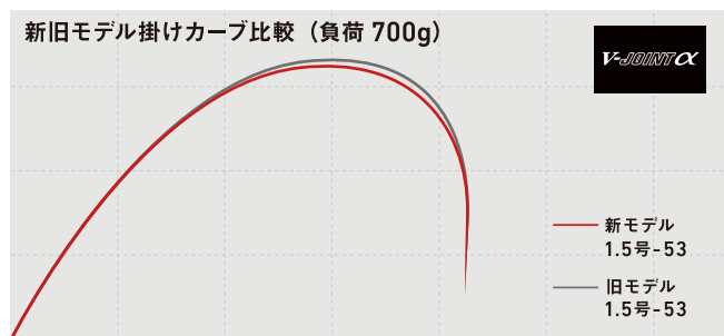
一定負荷において穂先はこの位置だが、さらに負荷が増すと、V-JOINT \alpha の効果でスムーズに節が張りすぎることなく曲がりこみ、急激な魚の引きに追従する調子となっている。
